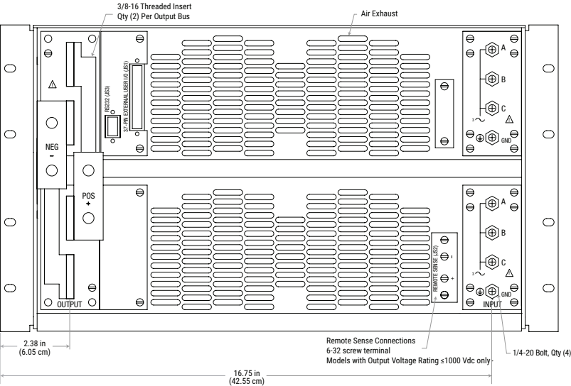
前面板 6U 型号
