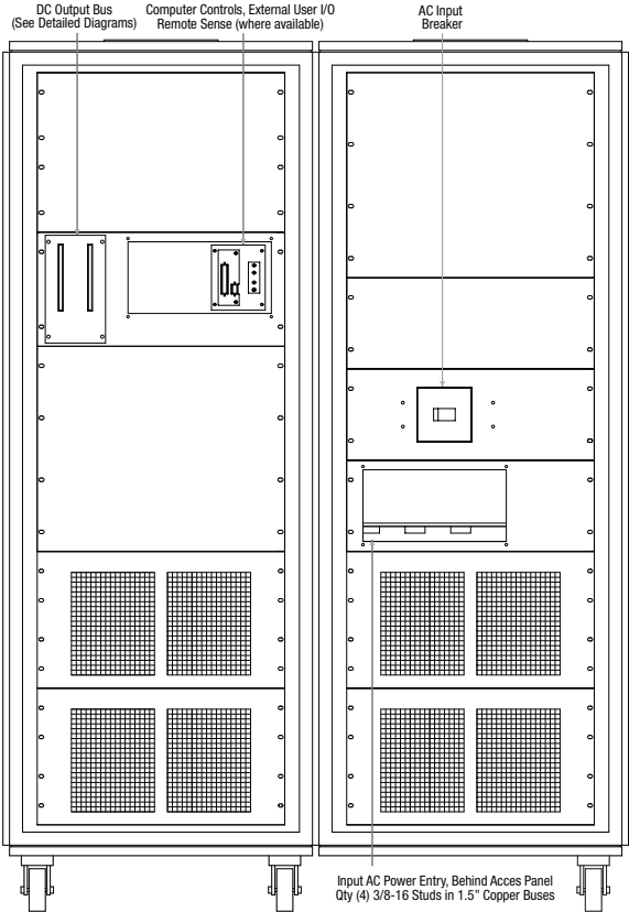
后侧 100 kW 和 150 kW 型号
