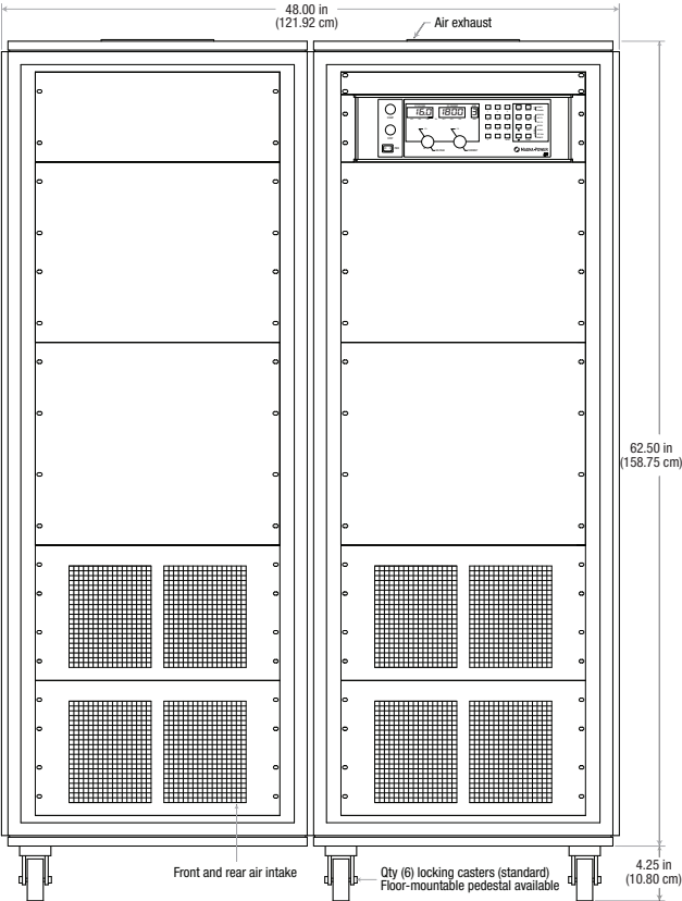
正面 100 kW 和 150 kW 型号
