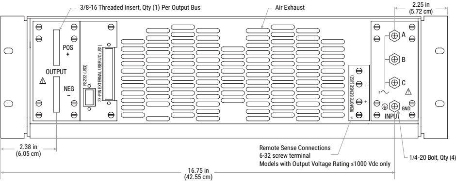
后面板 3U 型号
