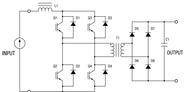
图2. 电流馈电式转换器
