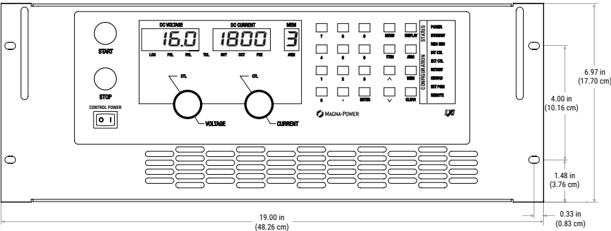
后面板 4U 型号
