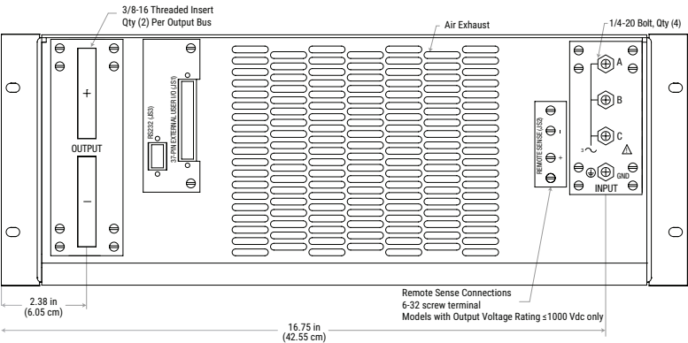
前面板 4U 型号
