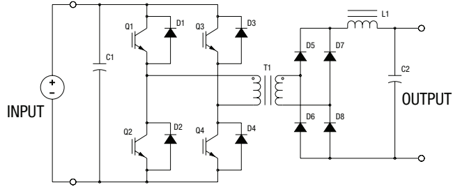
图1. 电压馈电式转换器
