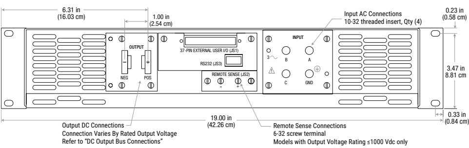
前面板
